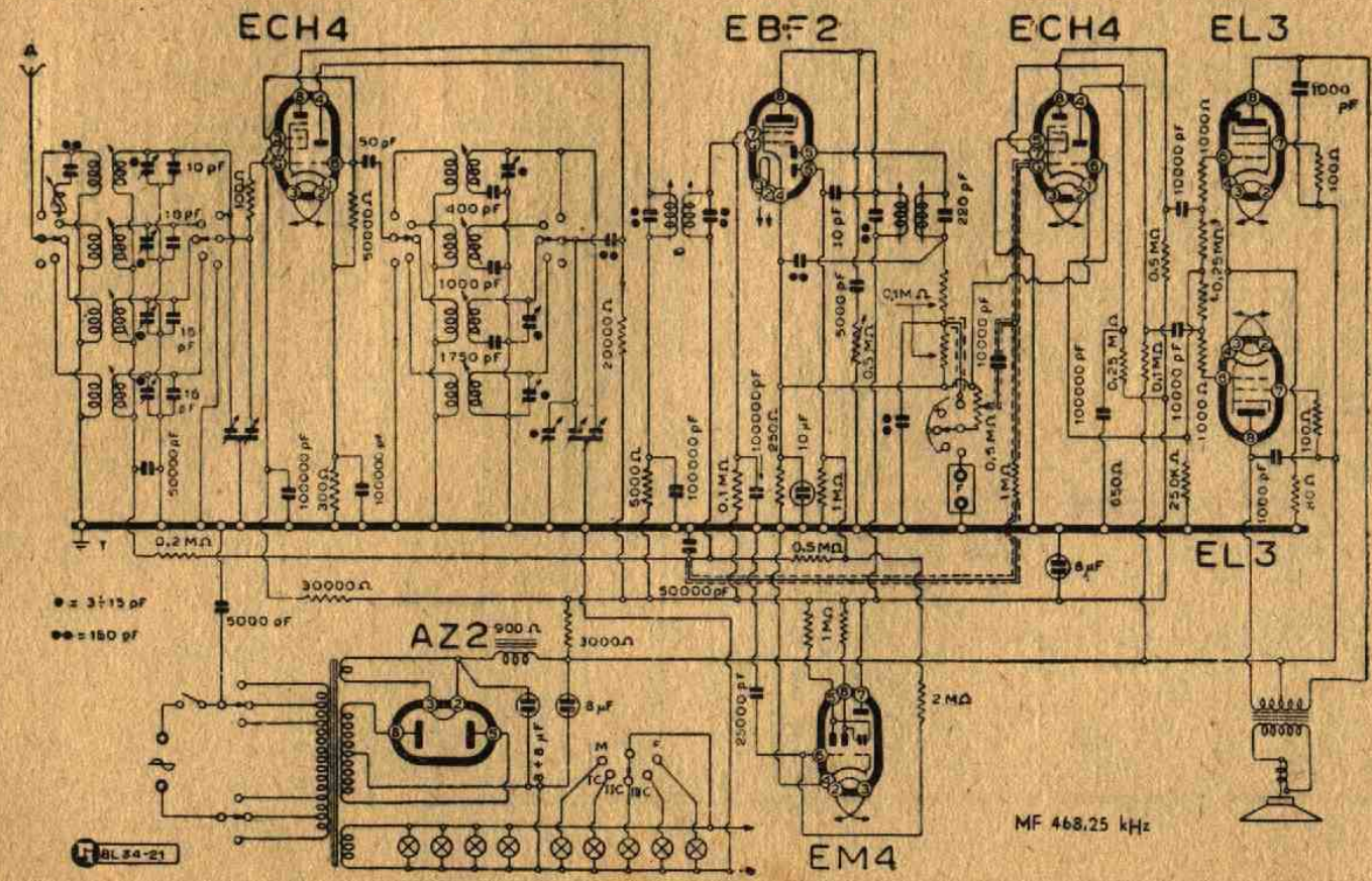
Lo schema elettrico del Superla mod. "647 B...
